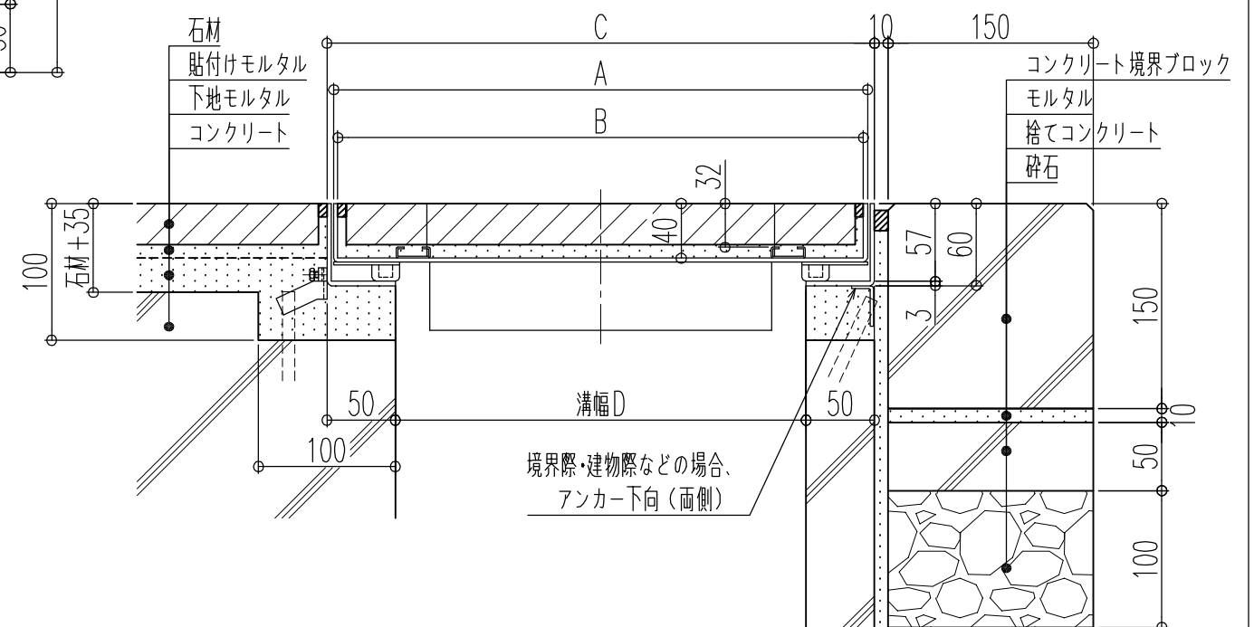
施工参考図
